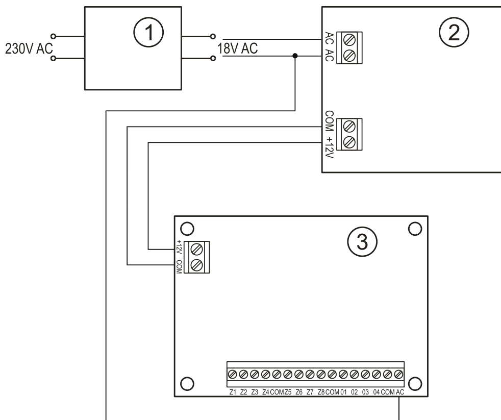
Rys. 4. Przykład podłączenia zasilania i kontroli obecności napięcia zmiennego w module GPRS-T4. 1 – transformator. 2 – zasilacz. 3 – moduł GPRS-T4.
