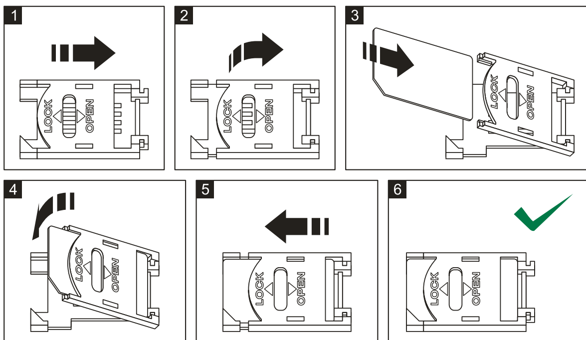
Rys. 5. Sposób montażu karty SIM.
