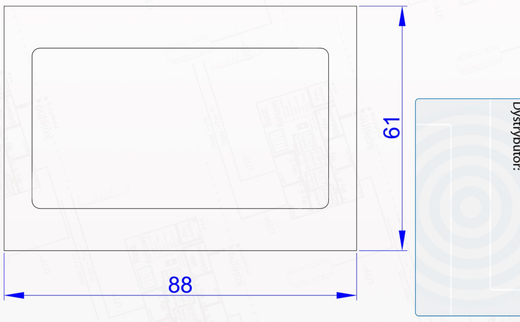
Wymiary modułu ACC
